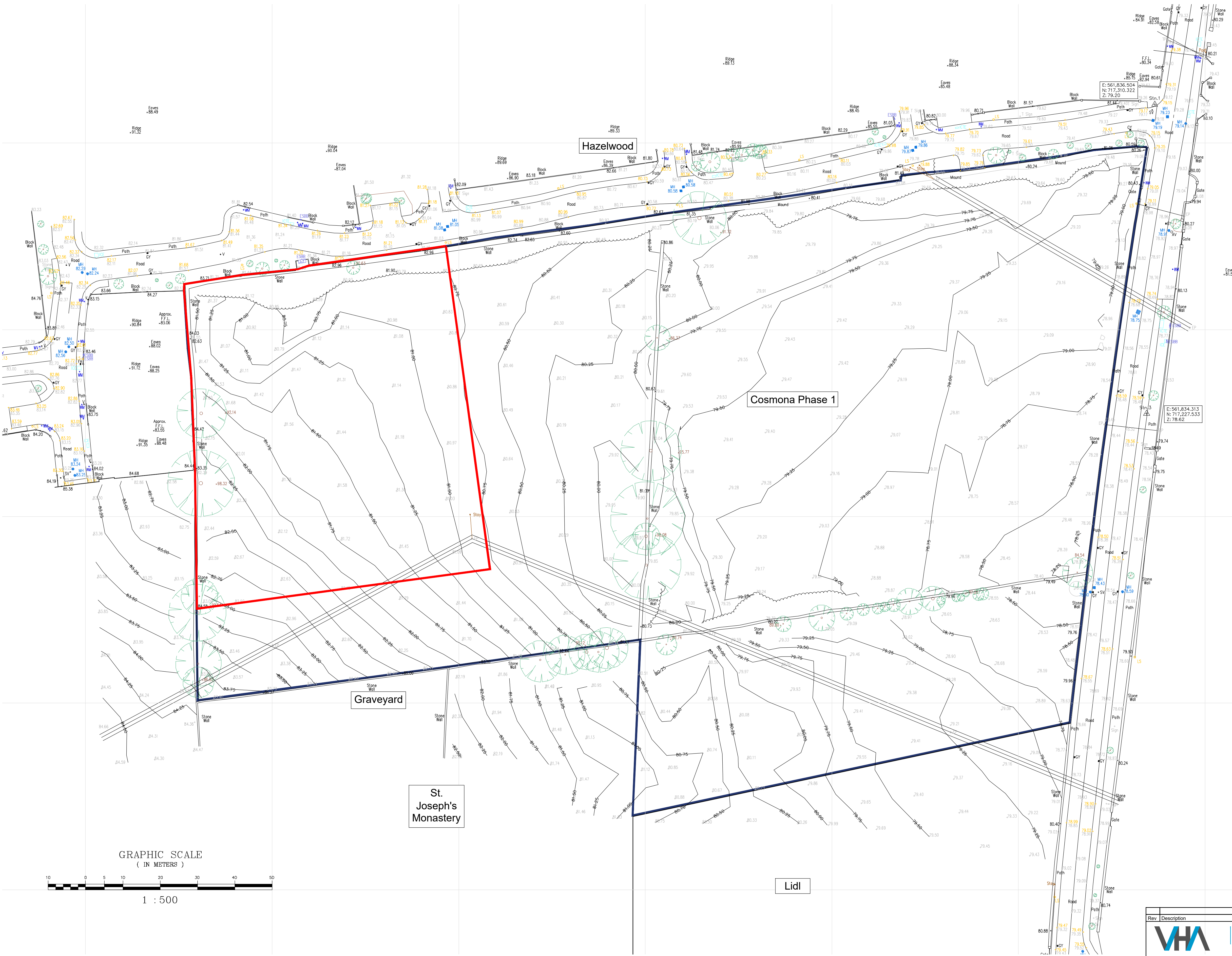
SITE SURVEY (Scale 1:500)
