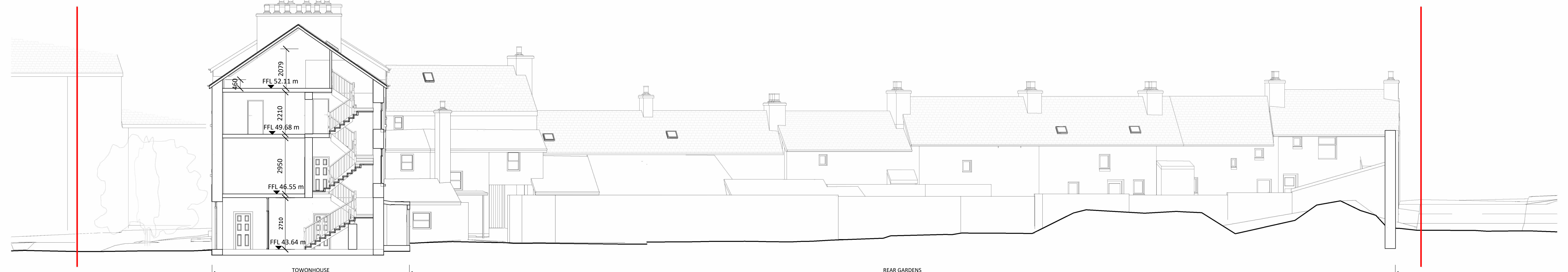
3 Existing Longitudinal Section C 1 : 100
