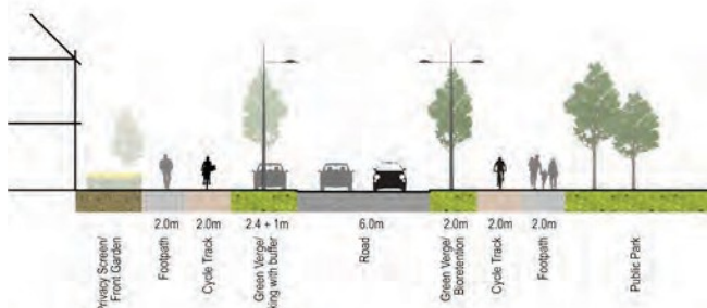
Príomhcheangal 2-2
