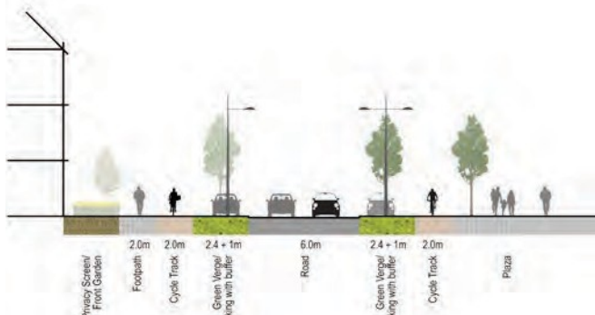
Príomhcheangal 1-1
