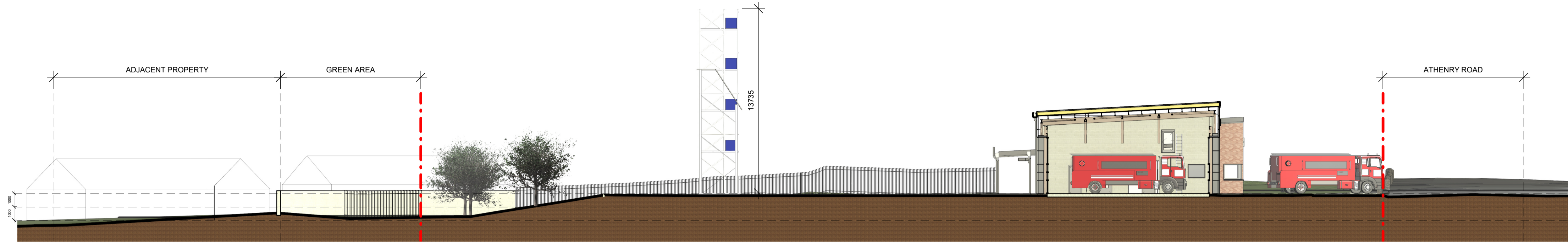
① Section A-A 1 : 200
